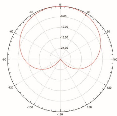
1520MHz-1615MHz
