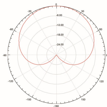
1164MHz-1300MHz
